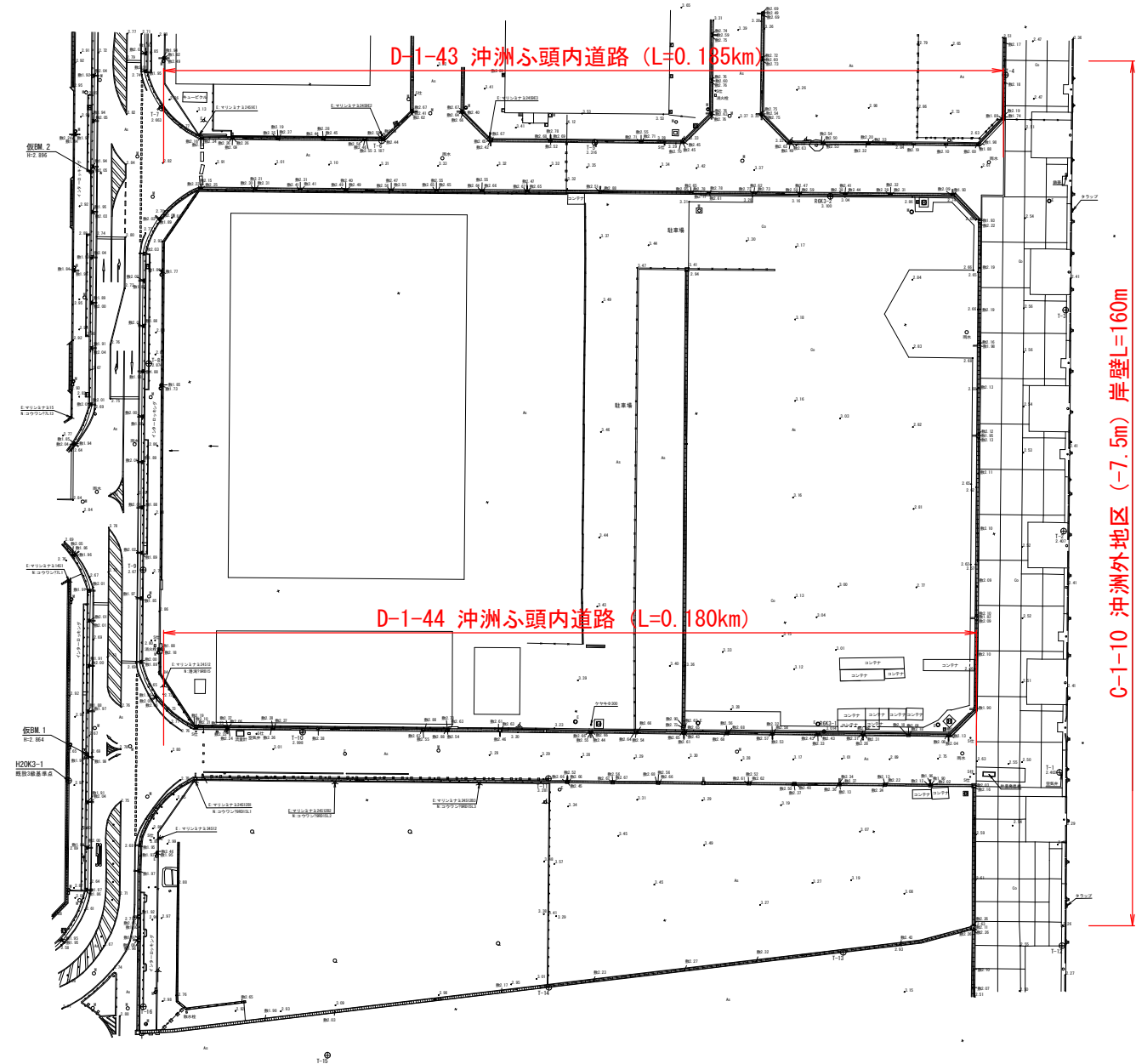
平面図 (対象施設)
